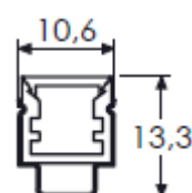
Profil avec clip
