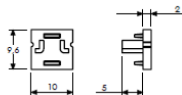
Clip de fixation
